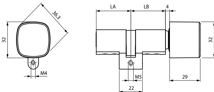
Kaba star Drehknopfzylinder, Typ M1519
